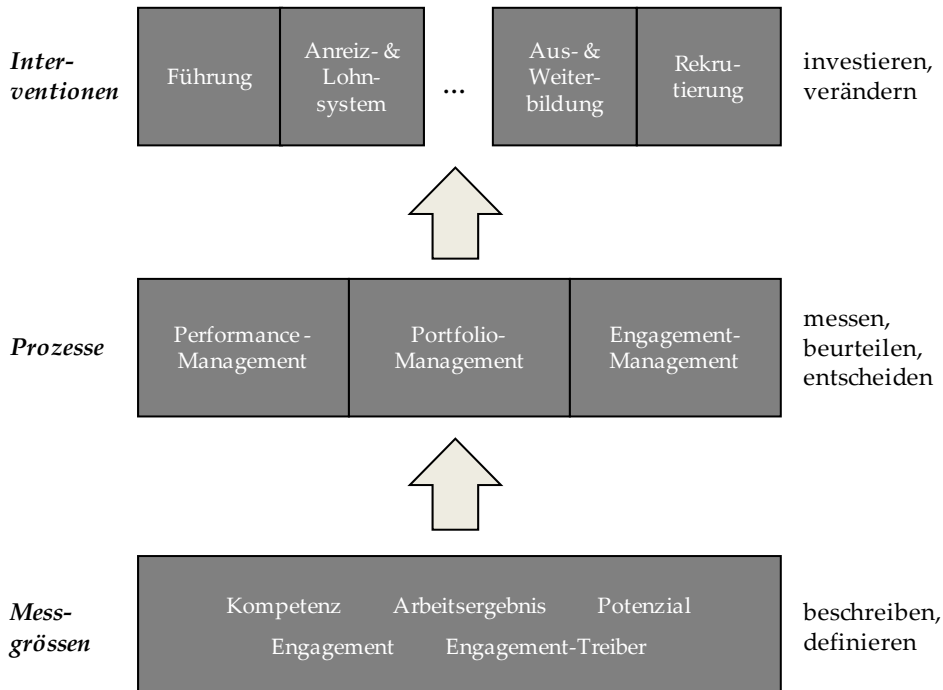
Abbildung 3.1 HCM-Architektur
